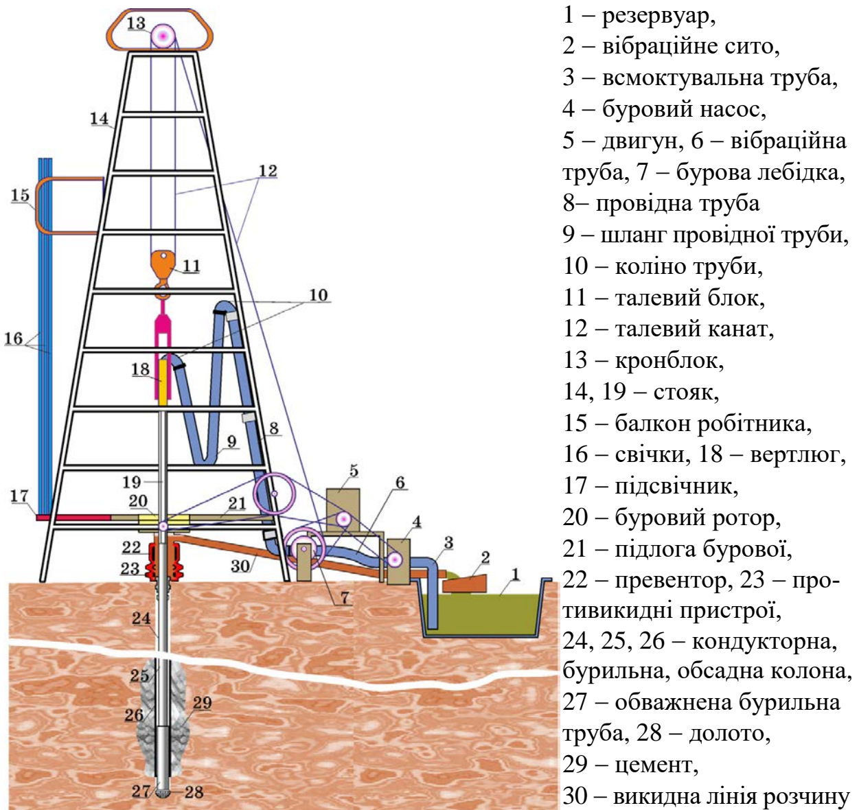
Рисунок 2 – Схема бурової установки
