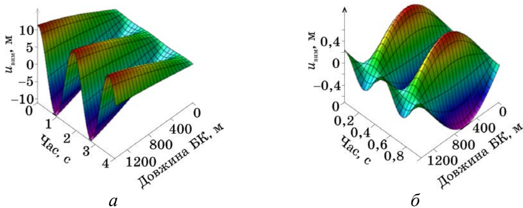
Рисунок 17 – Вимушені поздовжні коливання перерізів бурильних труб (біжучі хвилі), збурених поверхневим вібропристроєм, при налаштуванні на першу (а) і другу (б) власну частоту
