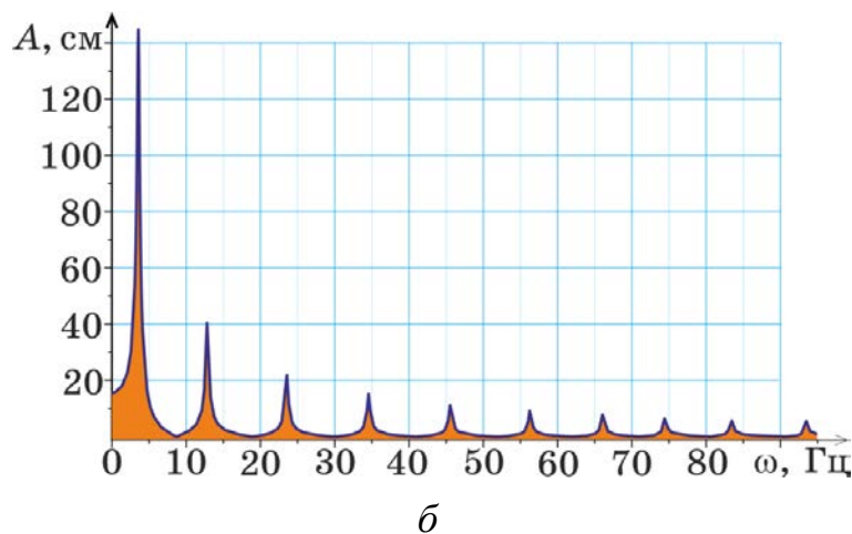
Рисунок 20 – Амплітудно-частотні характеристики коливальних систем бурильної колони з поверхневим осцилятором ( а ) для різних значень в'язкого опору і з глибинним вібратором ( б )
