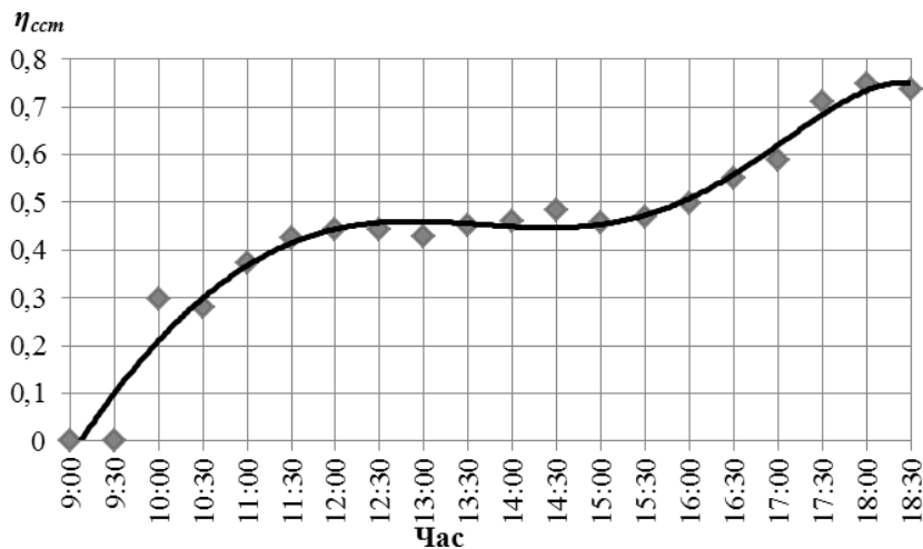
Рис. 7. Ефективність гравітаційної системи сонячного теплопостачання геліозахищення із геліовікном за умов південної орієнтації
