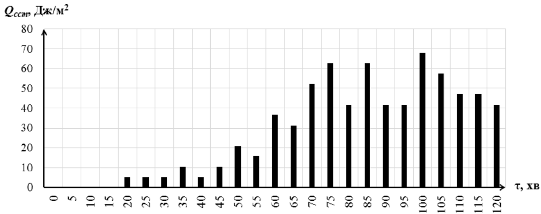
Рис. 4. Питома миттєва теплова потужність системи сонячного теплопостачання із геліостіною Q_{sst} , Дж/м 2 у режимі гравітації при I = 900 Вт/м 2
