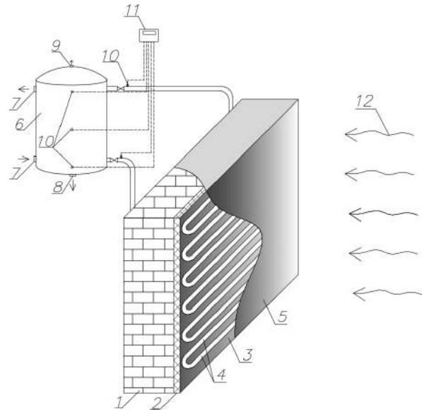
Рис. 1. Схема експериментальної установки: 1 – геліостіна; 2 – теплоізоляційний шар; 3 – тепловідбивний шар; 4 – трубки контуру циркуляції; 5 – тиньк; 6 – бак-акумулятор; 7 – патрубки відбору та надходження теплоносія; 8 – патрубок сливу теплоносія; 9 – повітровипускний клапан; 10 – термометри; 11 – дисплей; 12 – джерело випромінювання
